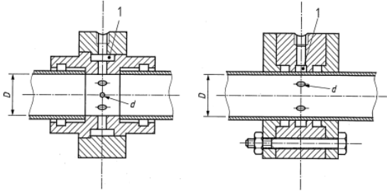
圖 2 鑽孔式測壓孔與其環室的範例 (適用於小/中直徑的量測段)
