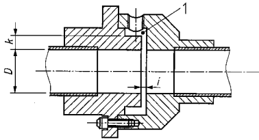
圖 3 環形槽測壓孔與其環室的範例 (適用於小/中直徑的量測段)
