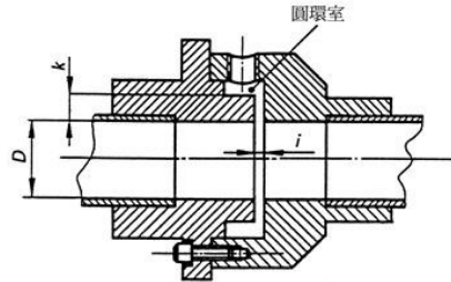
圖 A.5 開縫式測壓孔與其環室的範例 (適用於小/中直徑的量測段)
