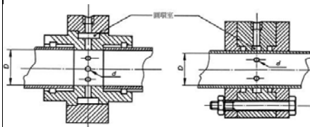
圖 A.4 鑽孔式測壓孔與其環室的範例 (適用於小/中直徑的量測段)
