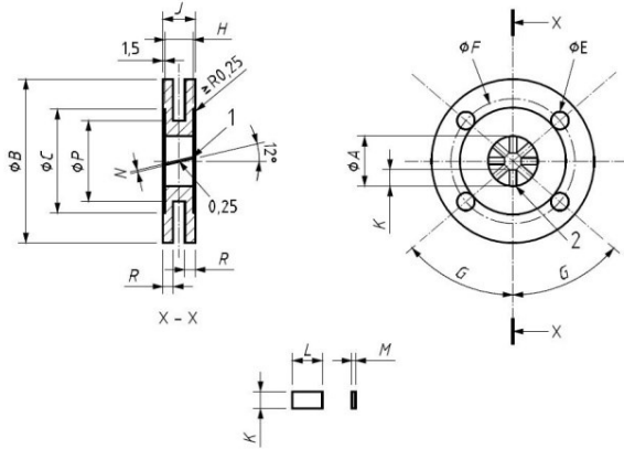
3 型干擾器：速度輪廓流動干擾器 圖 A.9 圓片式流場干擾器－速度輪廓干擾單元之配置
