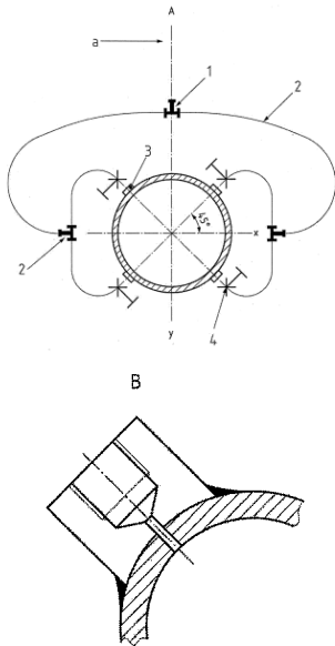
圖 3 環形槽測壓孔與其環室的範例 (適用於小/中直徑的量測段)
